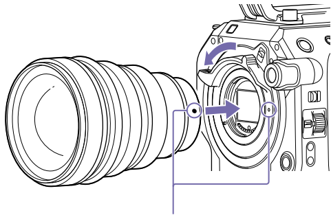
镜头座标记（白色）
